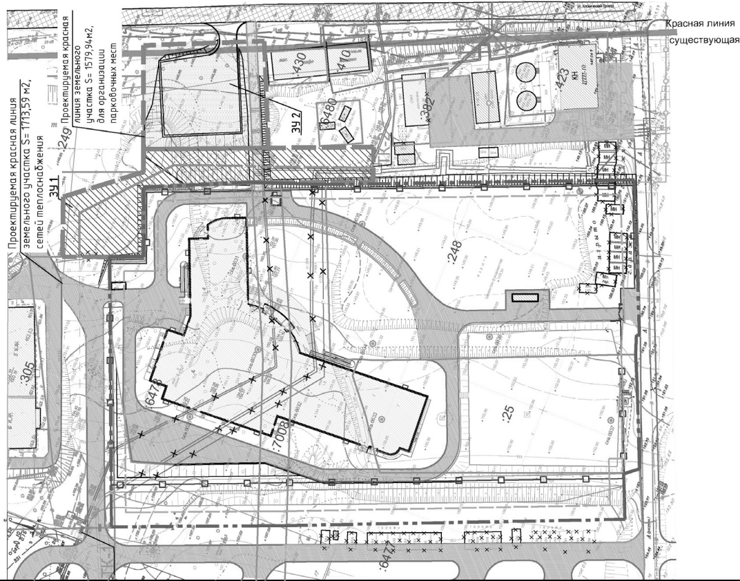
Схема границ зон размещения линейного объекта. М 1:1000
