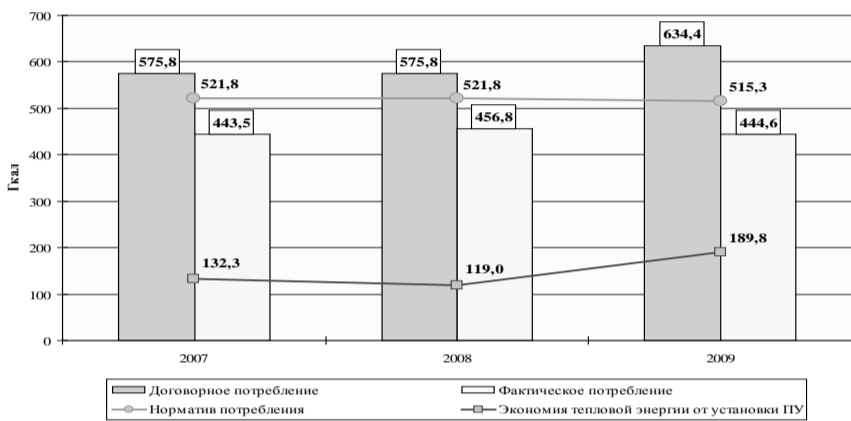
Анализ потребления тепловой энергии на отопление (Гкал) за 2007-2009 гг.
