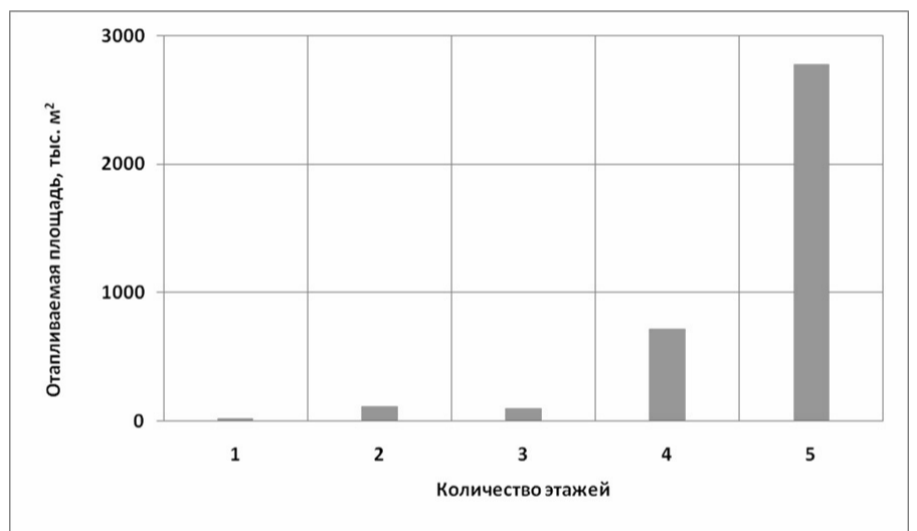
Рисунок 1.2 – Распределение отапливаемой площади по зданиям различной этажности
