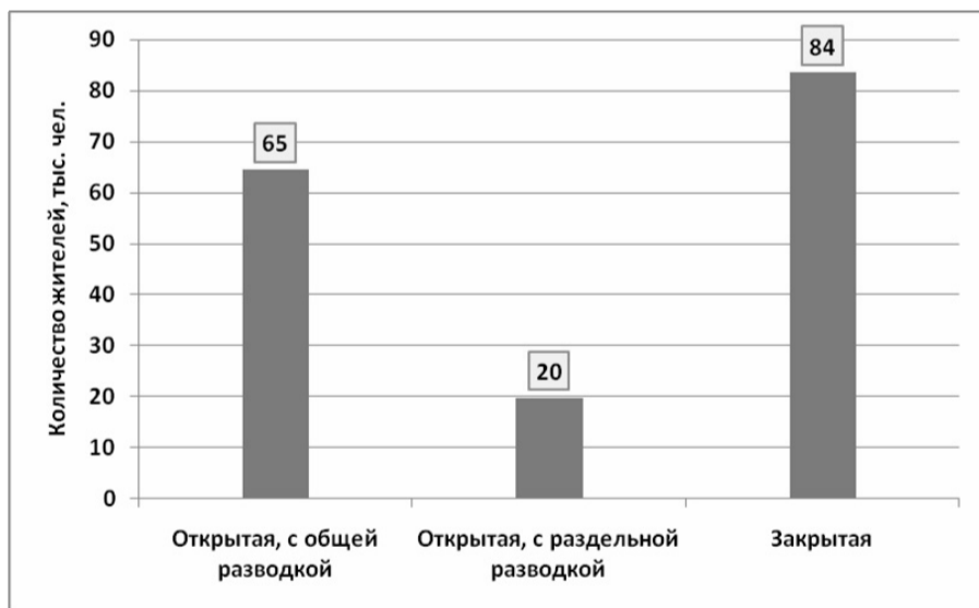
Рисунок 1.6 – Количество жителей и схема теплоснабжения зданий
