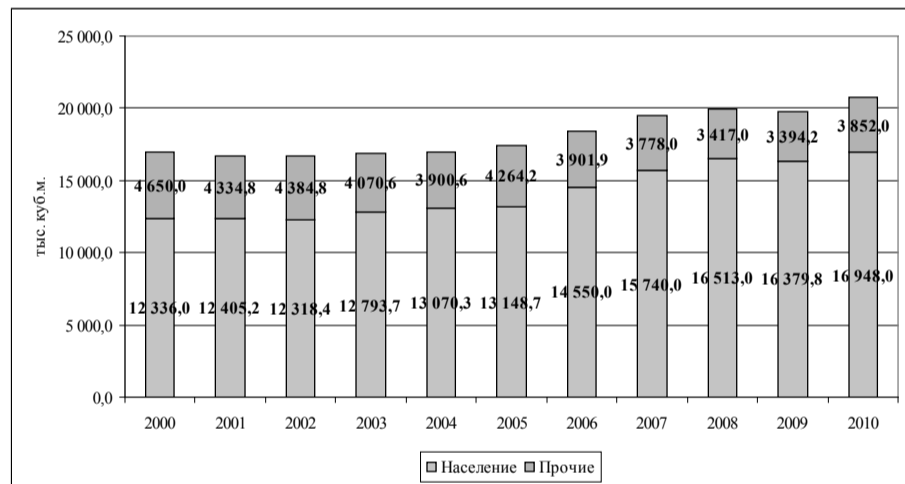
Рисунок 3.1 – Фактический объем предоставления услуг водоотведения по потребителям Петропавловск-Камчатского городского округа в 2000-2010 гг., тыс. м 3 .
