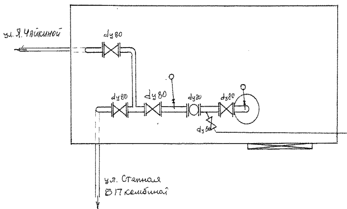
Рисунок 8 - Схема напорного трубопровода скв. «Степная»
