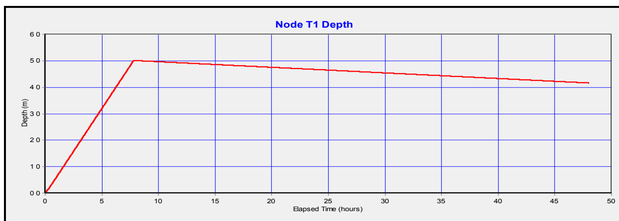
Рисунок 44 – Модельный график разгрузки приемного резервуара проектируемой КНС «Моховая», при поступлении расчетного результирующего расхода сточных вод 476 м 3 /ч, в том числе и от поселка Новый Новоавачинского сельского поселения
